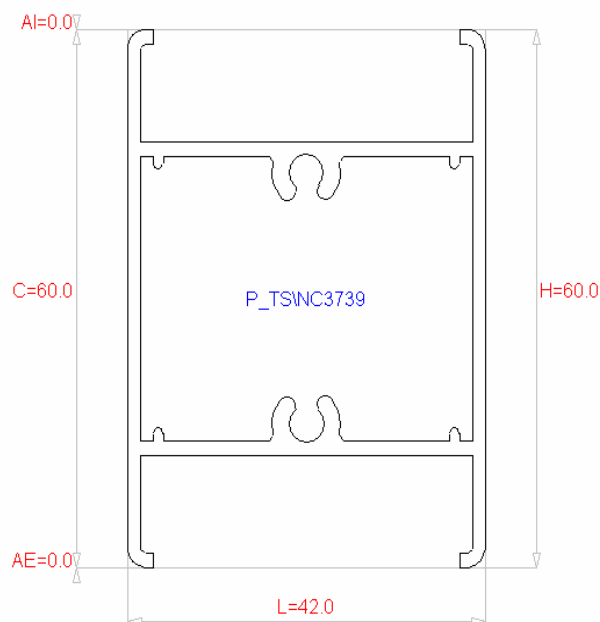
Traverso Portafinestre per esecuzioni SZ4B e SZ3B
