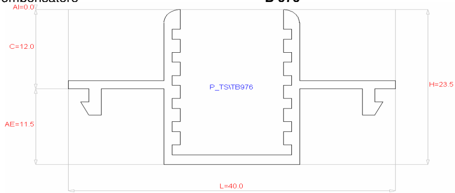
Riporto Centrale per Scambio Battute 2, 3 e 4 Ante
