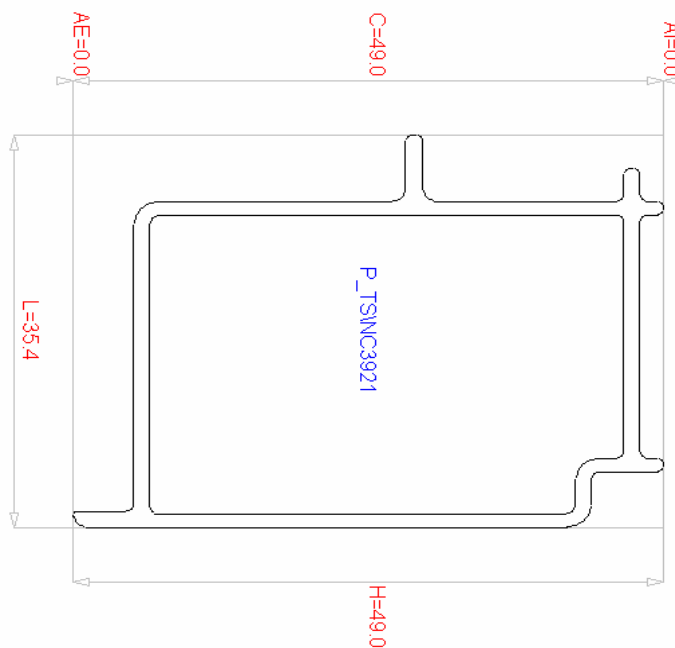
Riporto Centrale per Scambio Battute 2, 3 e 4 Ante
